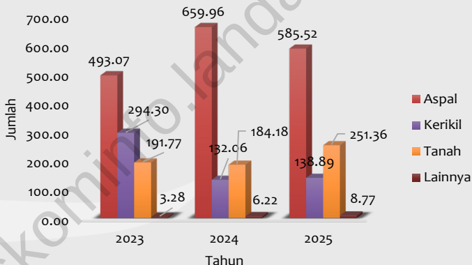
Grafik 8.2 Panjang Jalan Menurut Jenis Permukaan di Kabupaten Landak (Km) Tahun 2023-2025
