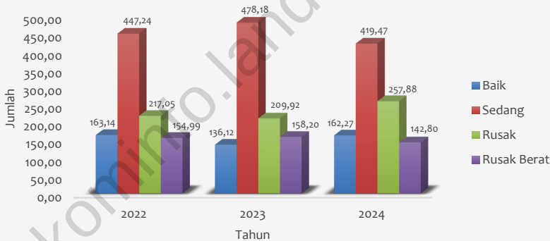
Grafik 8.3 Panjang Jalan Menurut Kondisi Jalan di Kabupaten Landak (Km) Tahun 2022-2024
